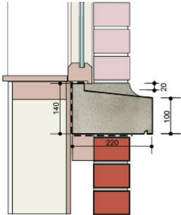
Section Dimensions 1:5
