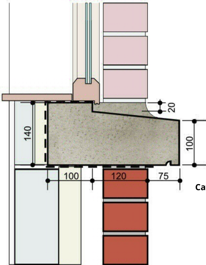
Section Dimensions 1:5
